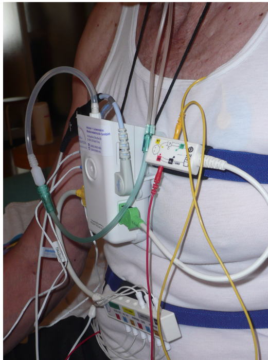
Abbildung 4 Aufzeichnungsgerät „Respironics Alice PDX“
